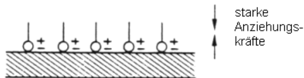
Kationische Tensidmoleküle auf einer Textiloberfläche
